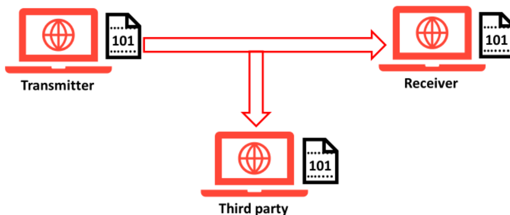
Abb. 1.1: Unbefugter Informationsgewinn
