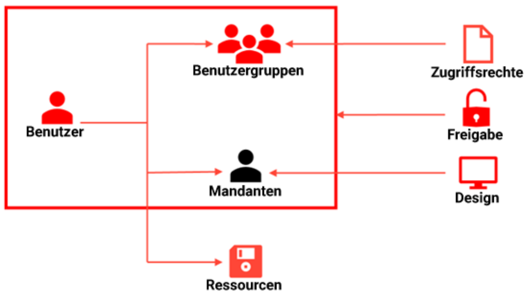
Abb. 3.1: Organisationsmodell
